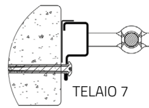
Telaio
